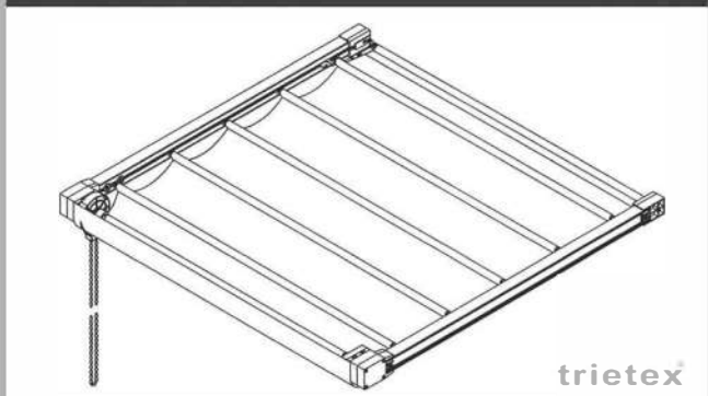
Zincirli Çatı Sistemi
