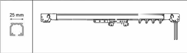
İpli Sistem (Çatı)
